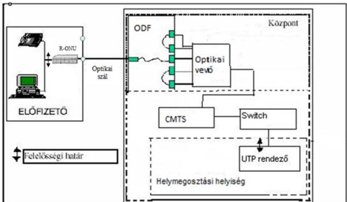
Közeli Bitfolyam Hozzáférés FTTH-RFoG Hozzáférési Hálózaton ábrája
