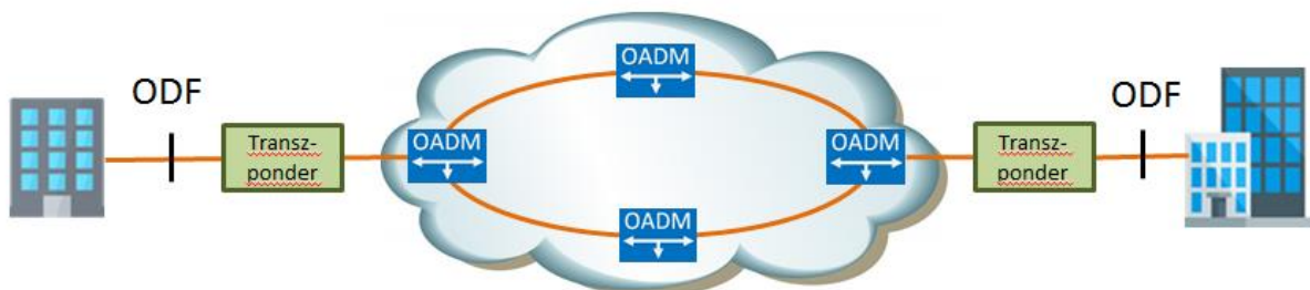
Gyűrű topológiájú WDM bérelt vonali hálózat
