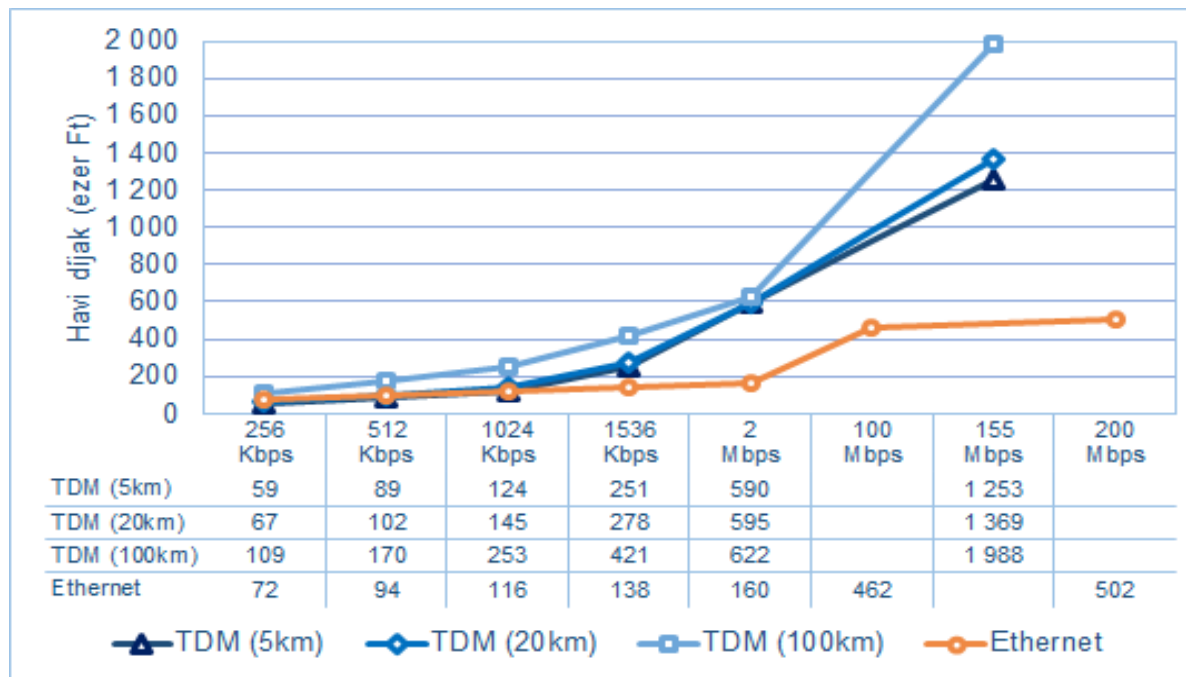
1. ábra: a Magyar Telekom TDM és Ethernet hozzáférések havi díjai
