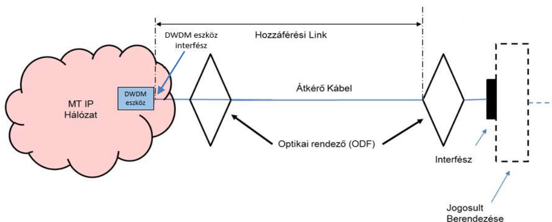
2. ábra: Hozzáférési Link szolgáltatás
