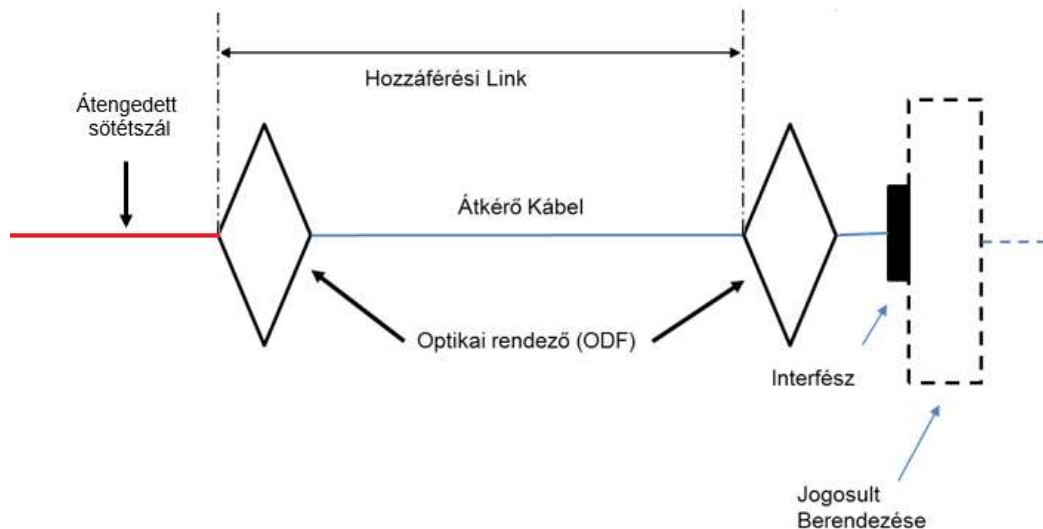
1. ábra: Hozzáférési Link Épületen belüli szakasz átkérő kábellel kiépítve
