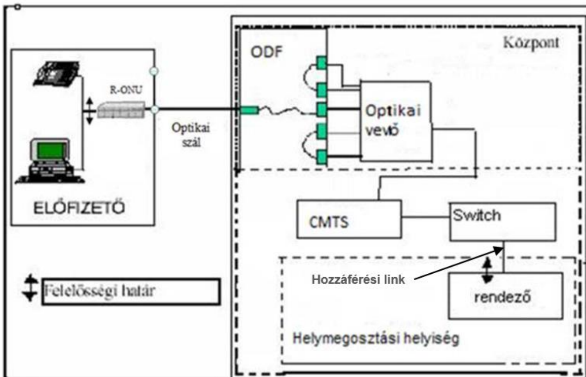
Közel Bifolyam Hozzáférés FTTH-RFoG Hozzáférési Hálózaton ábrája
