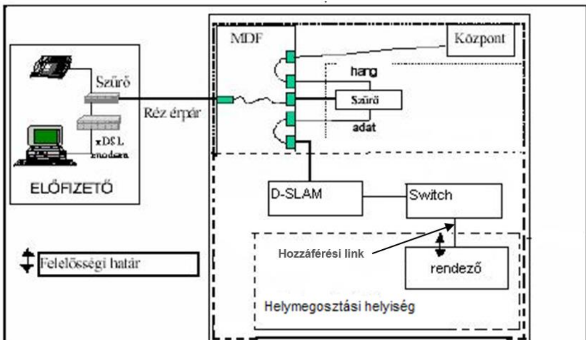
Közei bitfolyam hozzáférés réz érpáras hálózaton, helymegosztás esetén
