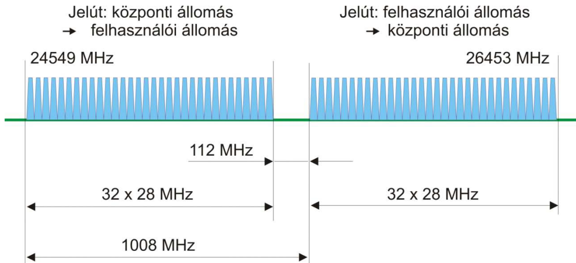
1. ábra A 26 GHz-es frekvenciasáv alaplókk felosztása
