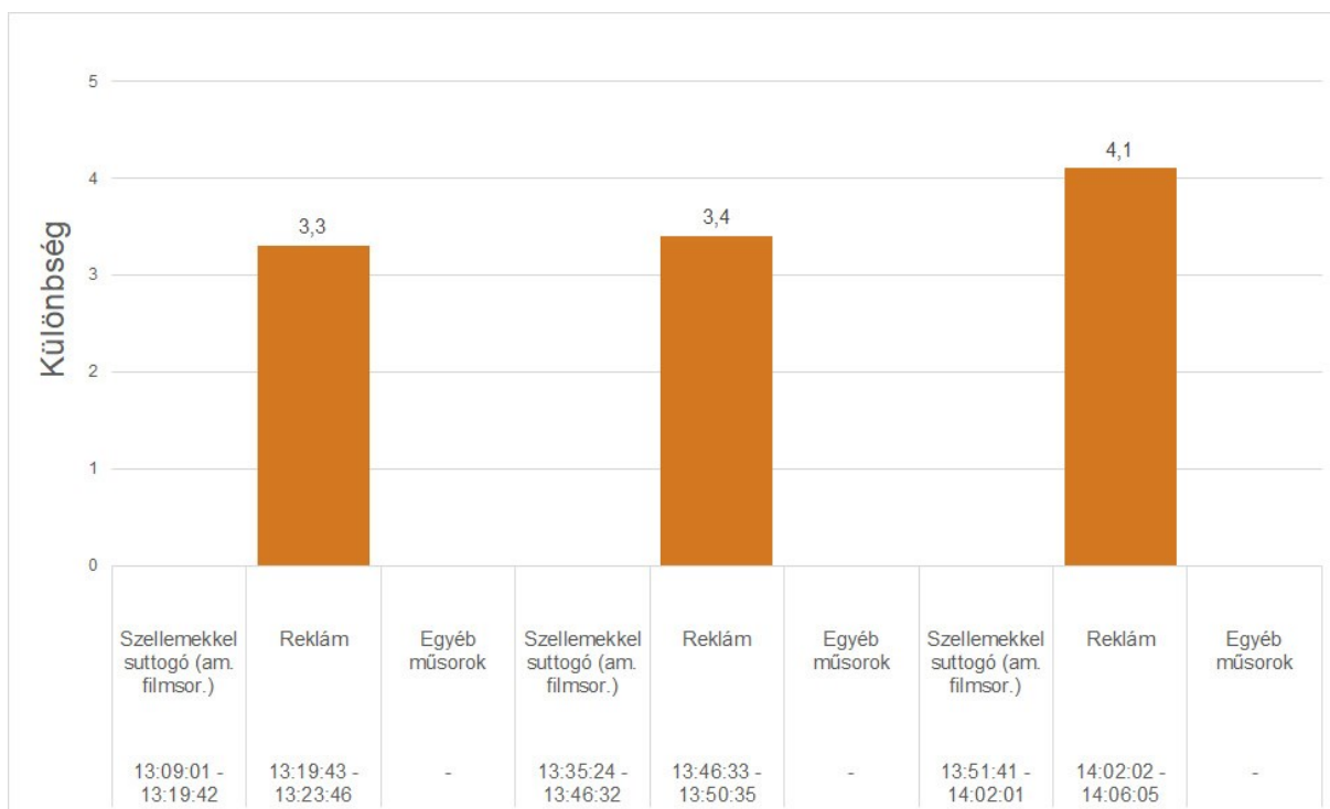
6. táblázat: Hangosságkülönbség-változás [dB] egymást követő műsorszámok esetén: Sonymax (2020. november 10.)
